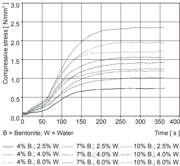
Figure 6. Graphical presentation of the measuring results for the mould mixture featuring granularity G2 Slika 6. Grafički prikaz rezultata mjerenja kalupne mješavine sa zrnatošću G2
