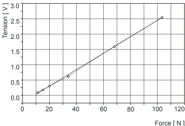
Figure 3. Calibrating diagram of the modified design of the compressive stresses gauge Slika 3. Baždarni dijagram modificirane izvedbe mjerilice tlačnih napetosti
