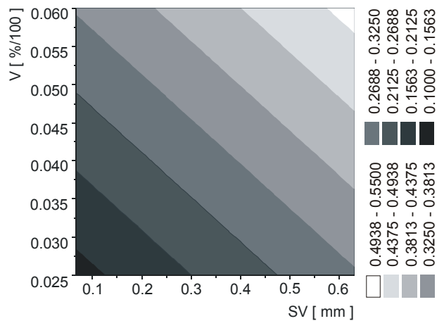
Figure 9. Regression model - contour plots Slika 9. Regresijski model - konturne plohe
