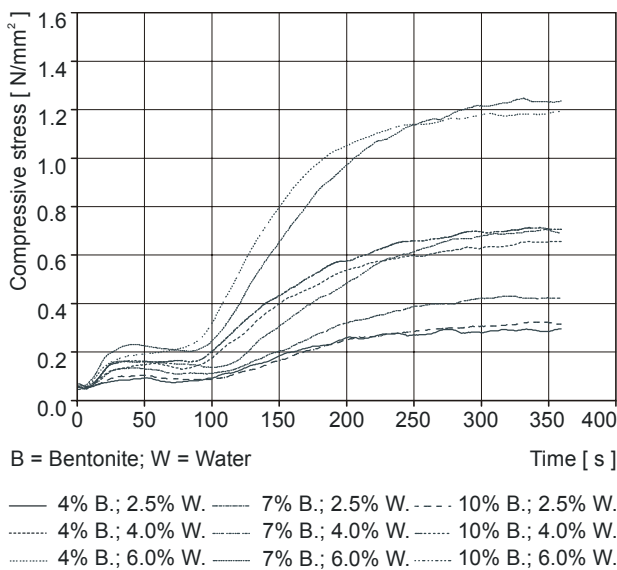
Figure 7. Graphical presentation of the measuring results for the mould mixture featuring granularity G3 Slika 7. Grafički prikaz rezultata mjerenja kalupne mješavine sa zrnatošću G3
