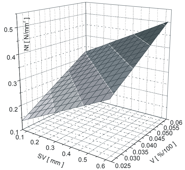
Figure 8. Graphical presentation of the regression model Slika 8. Grafički prikaz regresijskog modela
