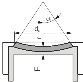
Figure 4. Test sample on the measuring apparatus Slika 4. Ispitni uzorak na mjernom osjetilu
