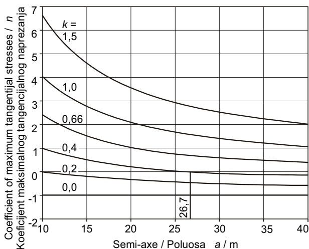
Figure 2. Dependence of the coefficient of maximum tangential stresses concentration in the roof of elliptical cross-section \sigma_{\text{an}}/k\sigma_v , at various character of primary state of stresses expressed by the coefficient k , on various value of the semi-axes a , (i.e. half span of the cavern) Slika 2. Ovisnost koeficijenta maksimalnog tangencijalnog naprezanja u svodu eliptičnog presjeka \sigma_{\text{an}} / \sigma_v pri različitim svojstvima primarnog stanja naprezanja izraženih koeficijentom k na različitim vrijednostima poluosi a (tj. pola raspona spilje)
