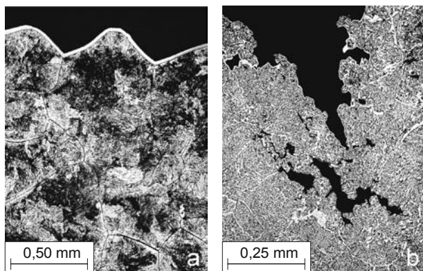
Figure 10. Intercrystalline fractures at the temperatures 900 a) and 1375 °C b), metallographic cross sections Slika 10. Medukristalni lomovi na temperaturama od 900 a) i 1375 °C b), medukristalni presjeci
