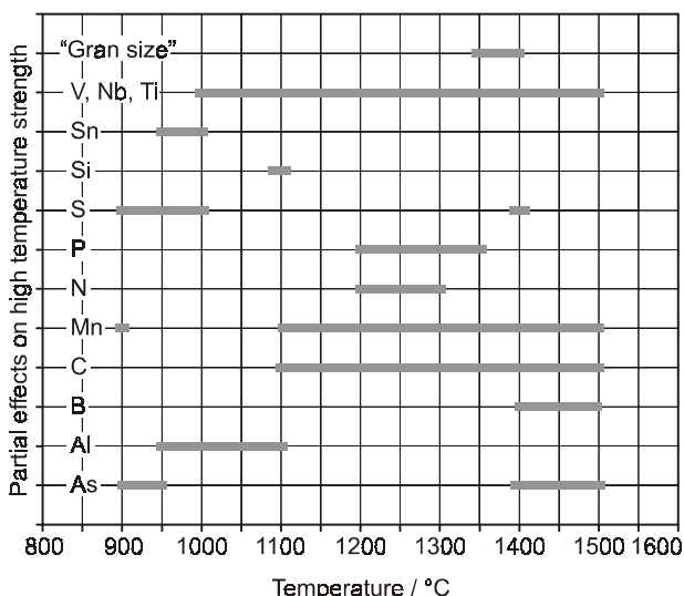
Figure 11. Schematic presentation of the influence of chemical composition and grain size on the high temperature strength Slika 11. Shematski prikaz utjecaja kemijskog sastava i veličine zrna na čvrstoću na visokoj temperaturi
