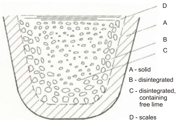
Figure 1. Disintegration of steelmaking slag after addition of crushed limestone into slag ladle Slika 1. Razlaganje čeličanske troske nakon dodavanja usitnjelog vapnenca u lonac s troskom
